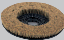
Bassine-Bürste für leichte Verschmutzungen ø 330 mm für S 35 E / S 35 B Bestell-Nr.: 5941005 ø 450 mm für S 45 E / S 45 B Bestell-Nr.: 5941006 ø 500 mm für S 50 E / S 50 B Bestell-Nr.: 5941007
