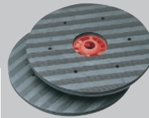
Treibteller mit Haftstreifen für Pads ø 330 mm für S 35 E / S 35 B Bestell-Nr.: 5941015 ø 450 mm für S 45 E / S 45 B Bestell-Nr.: 5941016 ø 500 mm für S 50 E / S 50 B Bestell-Nr.: 5941017
