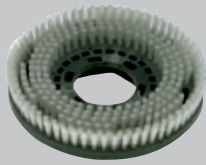
Polypropylene-Bürste für normale Verschmutzungen ø 350 mm für S 35 E / S 35 B Bestell-Nr.: 5941001 ø 450 mm für S 45 E / S 45 B Bestell-Nr.: 5941002 ø 500 mm für S 50 E / S 50 B Bestell-Nr.: 5941003
